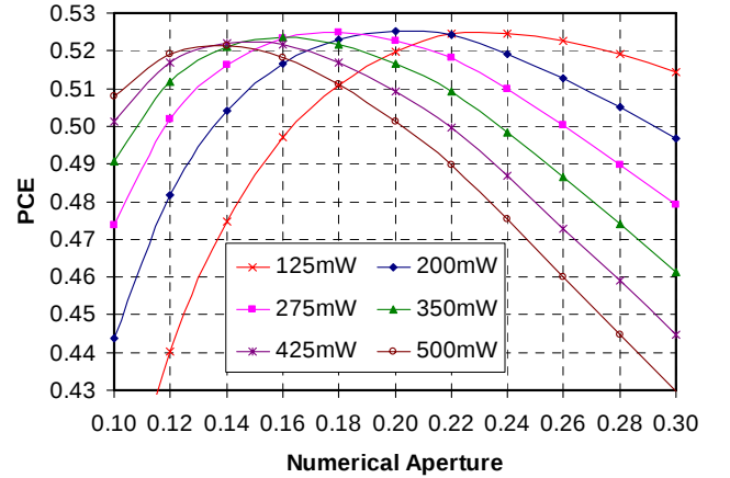
Fig. 2 PCE vs. NA
